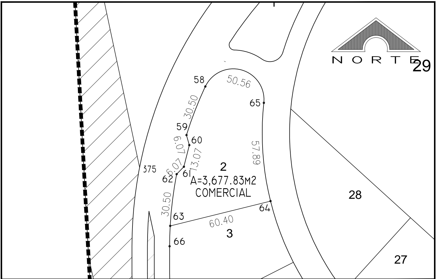
CUADRO DE CONSTRUCCION LOTE 2 MANZANA 2
